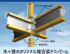
木+鉄のオリジナル複合梁テクノニーム
